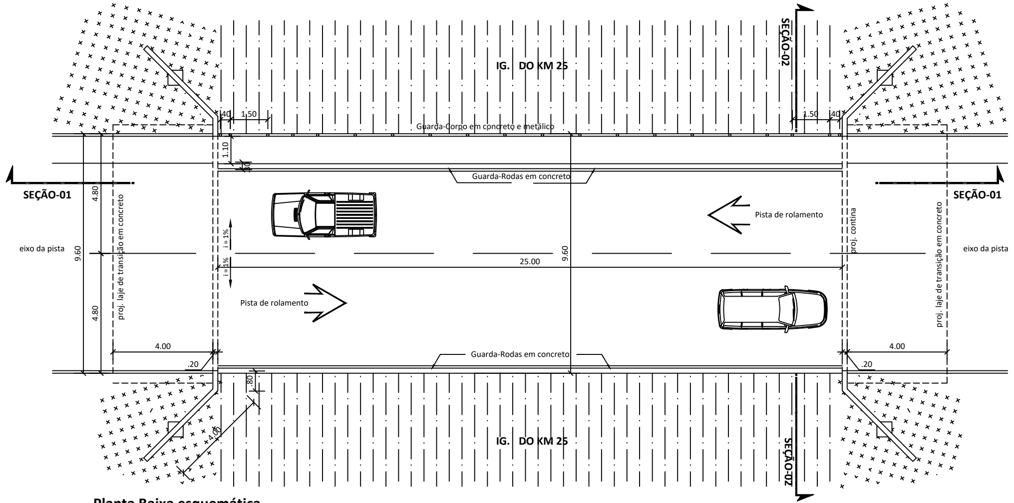
Planta Baixa esquemática
